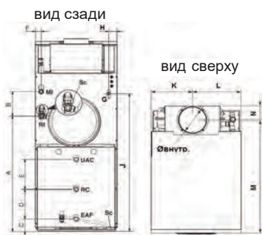
Fabula 35E-43E/120
