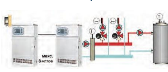
Каскадная установка
