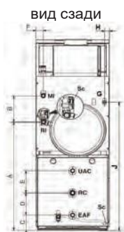
Fabula 27E-35E-43E/90
