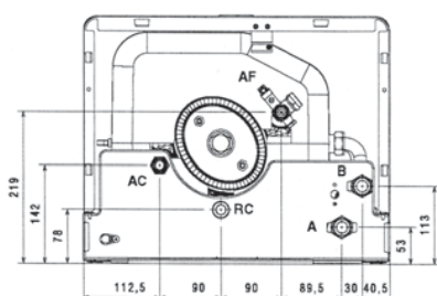
ВИД СНИЗУ
